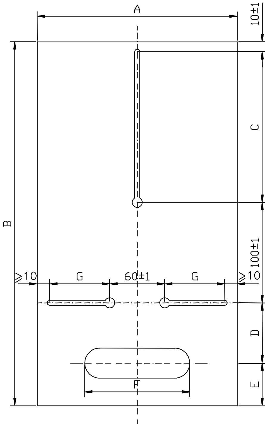
Figura 2 Placa soporte contadores
